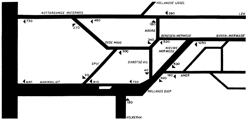
Fig. 5 De afvoerverdeling over het benedenrivierengebied bij een Bovenrijnafoer van 1500 m³/sec. bij toestand T 0 (boven) en toestand T 1 (beneden). De Haringvlietssluisen zijn dicht. Op Spui en Dordtse Kil veranderen de stromen van richting
