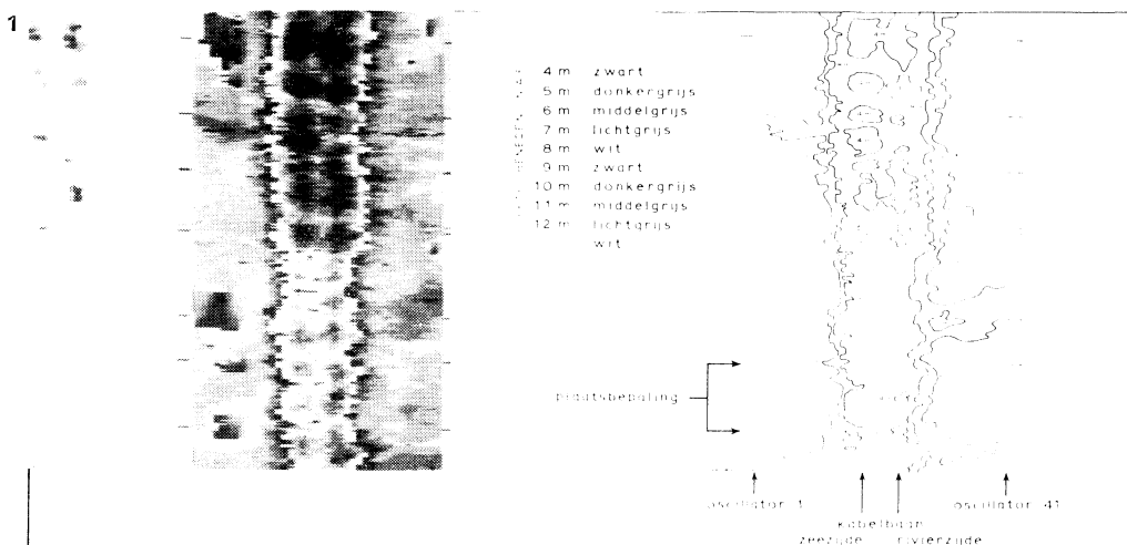
Fig. 1 Een registratie van de hoogteligging van de damkruin in het Rak van Scheelhoek, verkregen met het peilschip 'Krabbe', op 14 februari 1970
