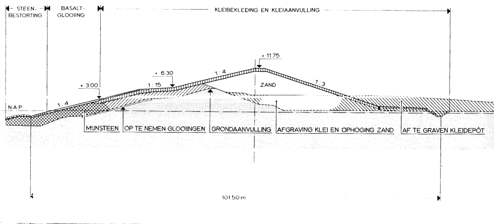
Dwarsdoorsnede A
