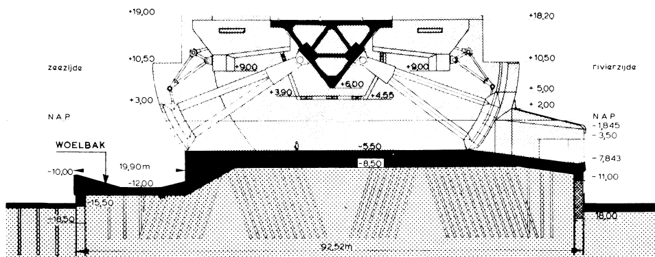
DWARS DOORSNEDE
