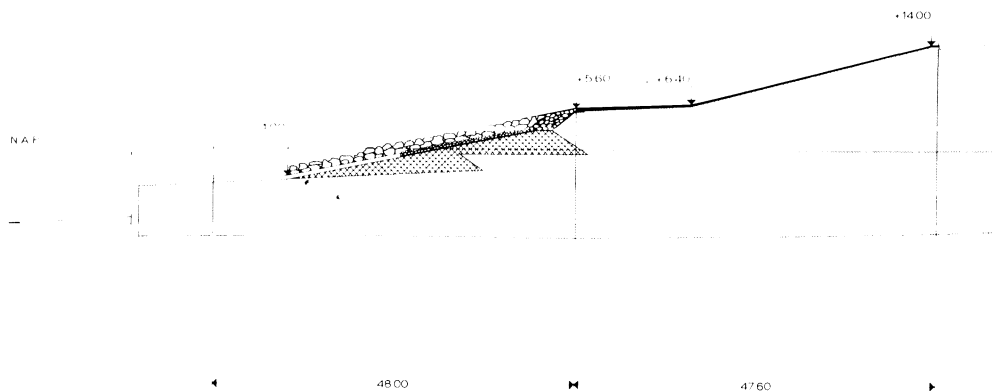
Fig. 3 Normaal dwarsprofiel van de oeeververdediging
