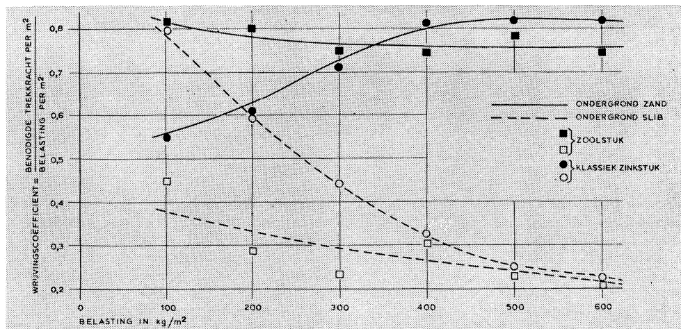
Fig. 2 Verloop van de wrijvingscoëfficiënt van een zoolstuk en een klassiek stuk over verschillende ondergrond bij toenemende belasting
